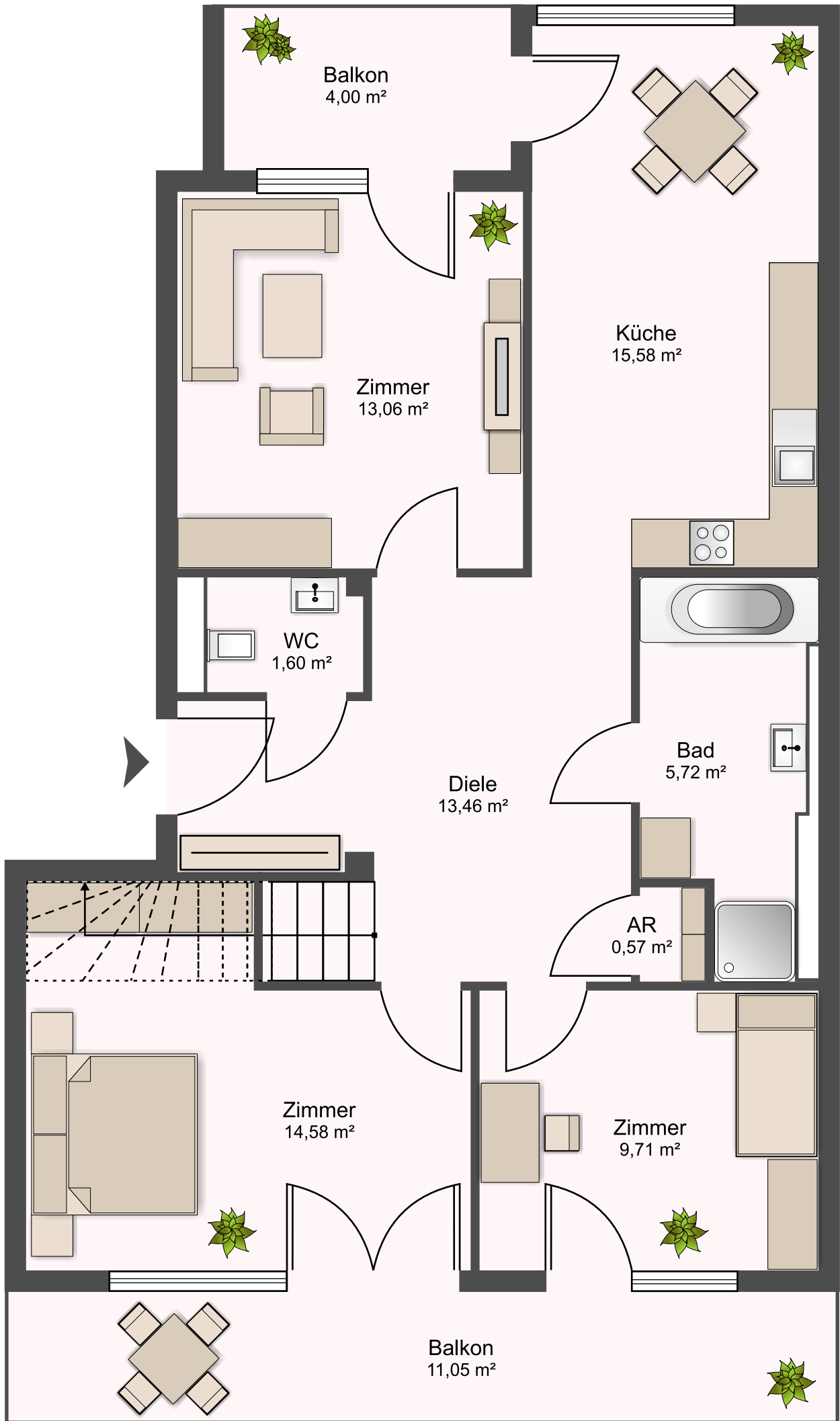
3. Obergeschoss
