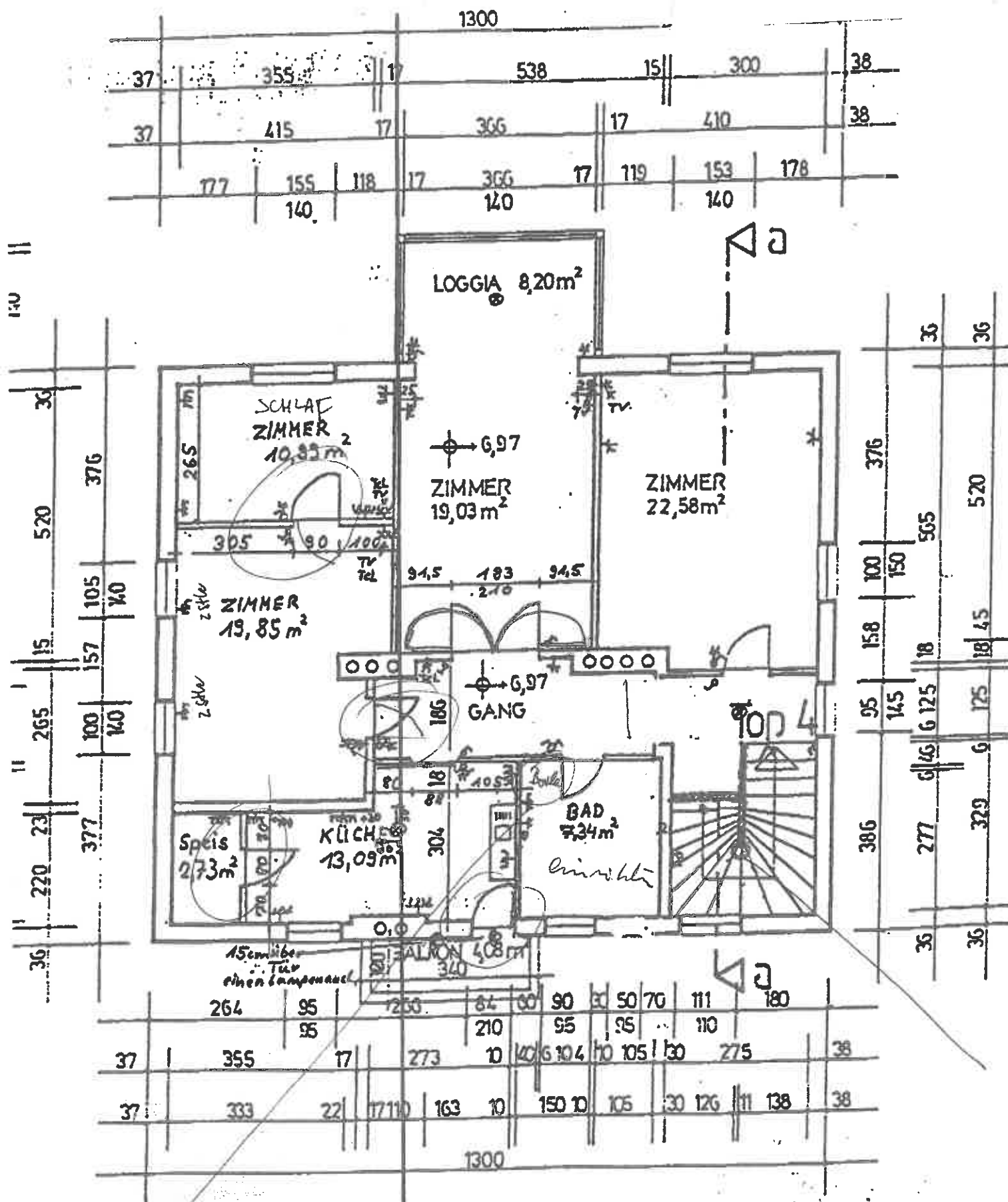
2. Obergeschoßgrundriß Top 4
