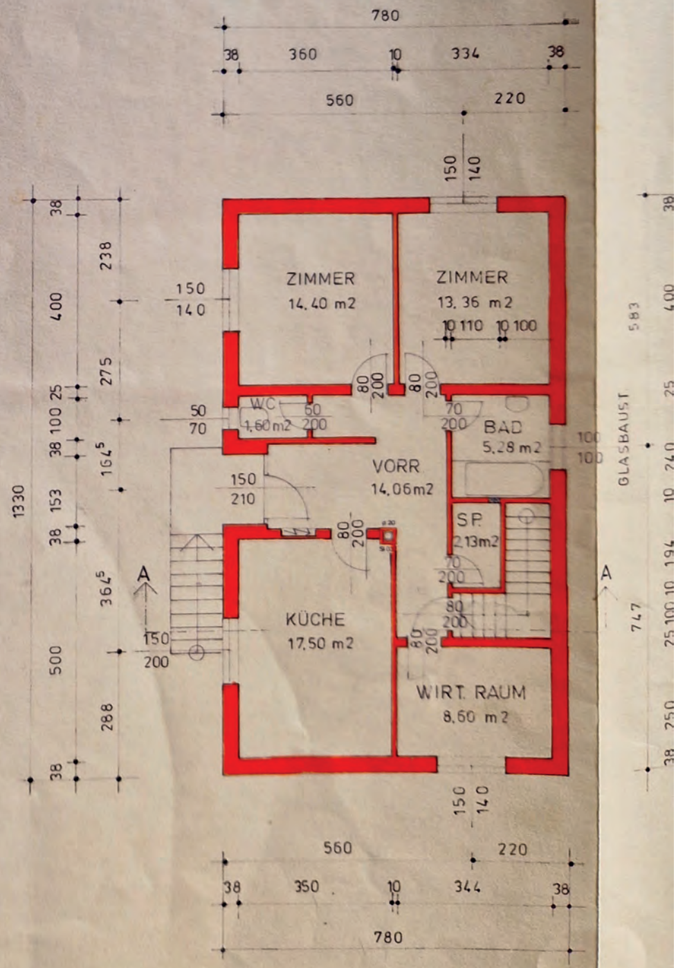
ERDGESSCHOSS
