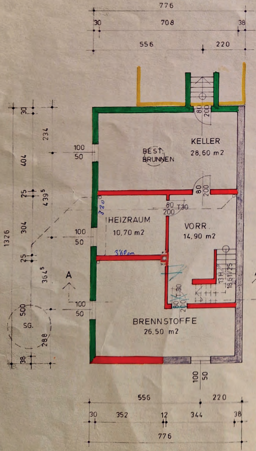
KELLERGESSCHOSS
