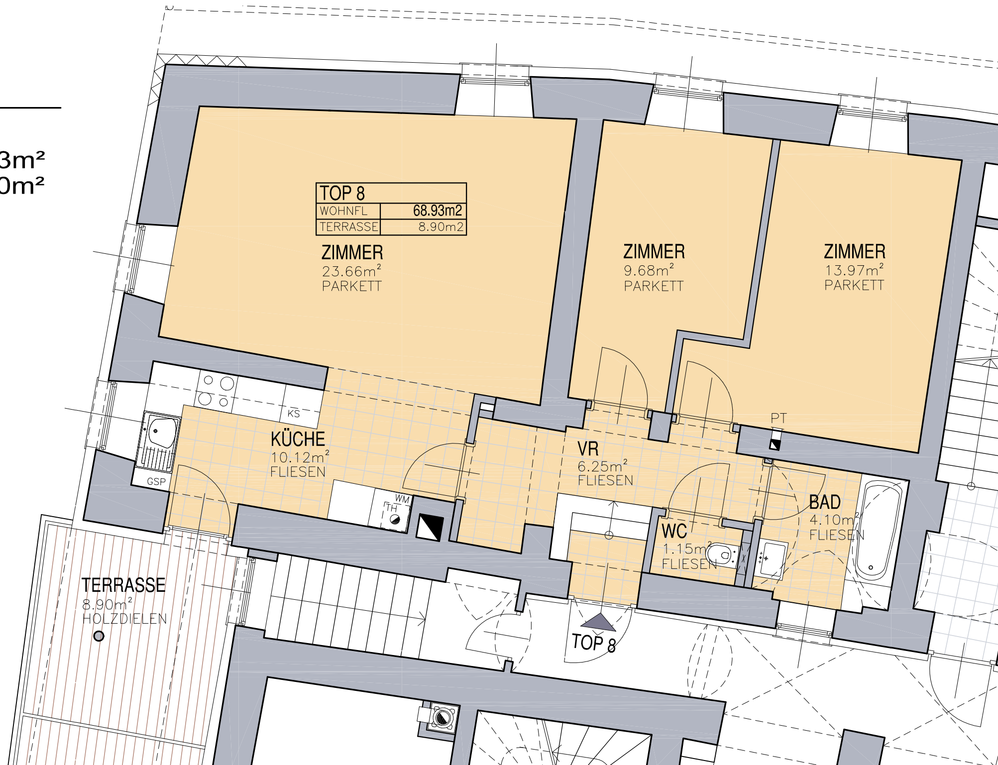
GRUNDRISS ERDGESCHOSS
